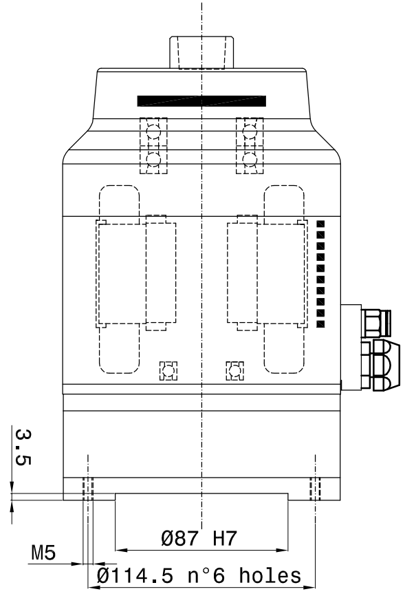
ARBOR HSK-E32 DIN 69893
