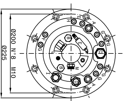
TOOLHOLDER HSK-A/E-50/63 DIN 69893
